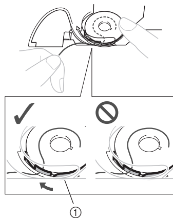
① Napínací pružinka
